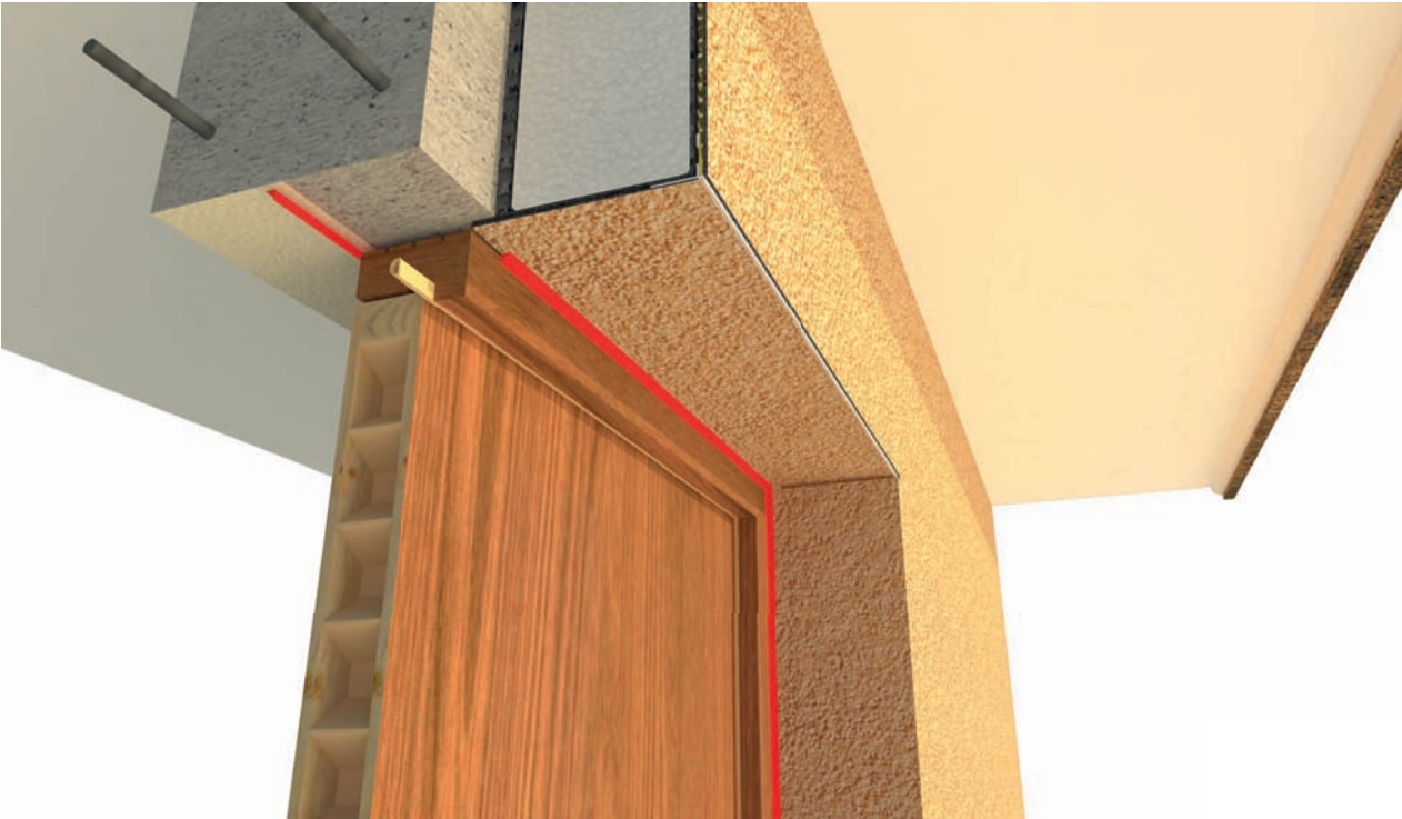
DETALLE 1
