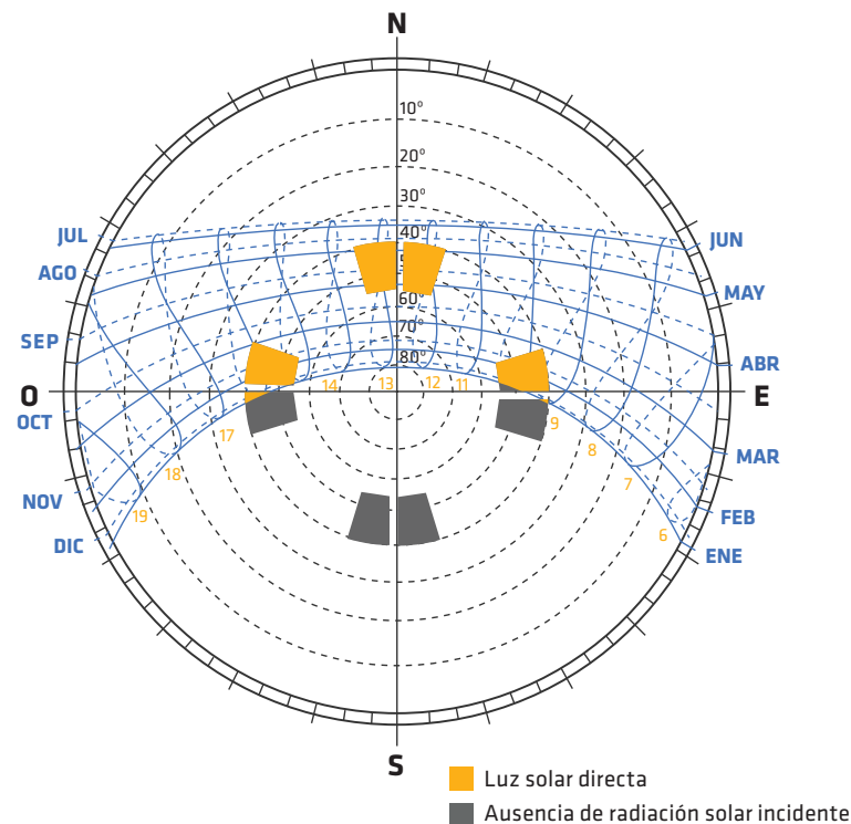
Figura III.3.4.2.5: Carta solar de proyección estereográfica para Valparaíso y Santiago. Accesibilidad a la luz solar directa en recinto tipo de vivienda social (3,6 x 2,8 m) a través de una ventana de 1,0 x 1,0 m en las distintas orientaciones
