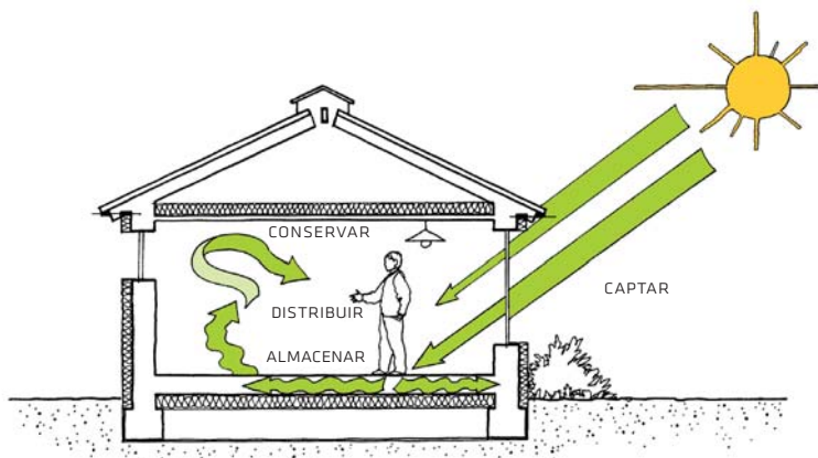
Figura II.1.1: Estrategias generales para periodos de frío.
