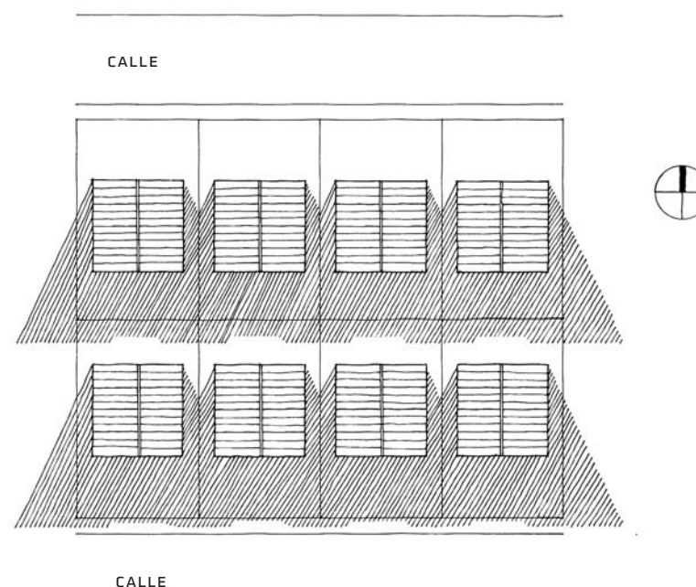
Figura III.2.1.2.1: Calles en sentido oriente poniente permiten acceso solar en fachada norte.
