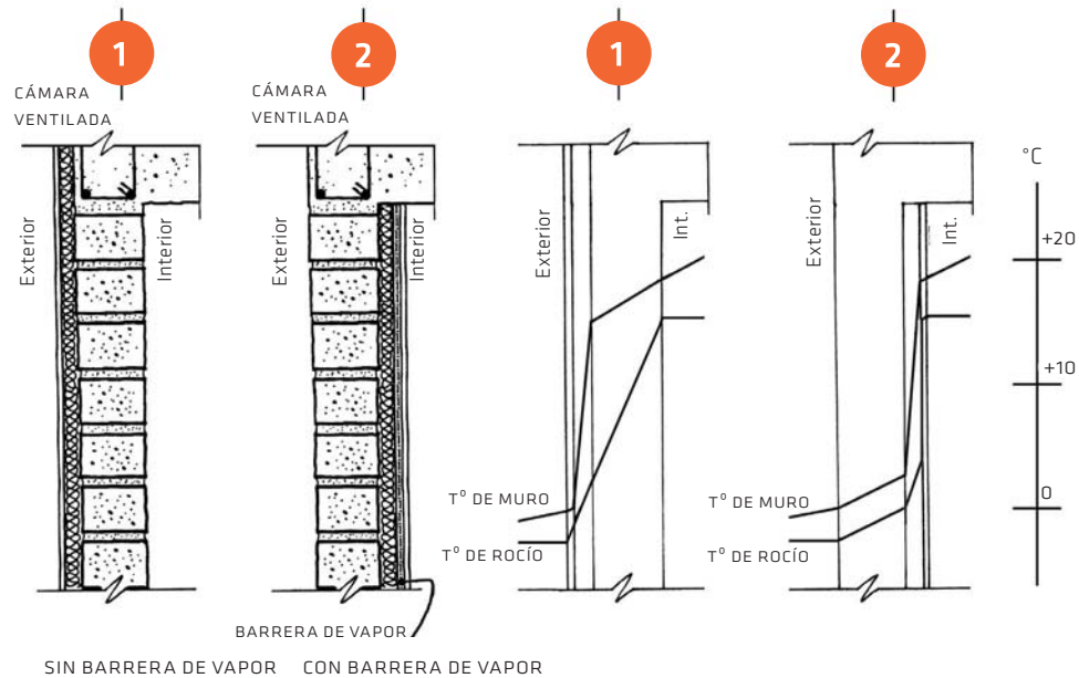
Figura III.3.8.2.4: Riesgo de condensación superficial e intersticial en muro de albañilería con 70mm aislación térmica exterior (1) y 70mm de aislación térmica interior (2).
