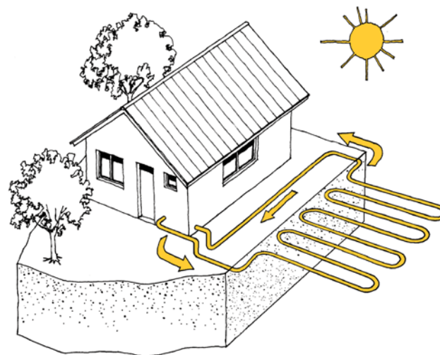
Figura IV.4.1: Sistema de intercambio de calor con subsuelo.
