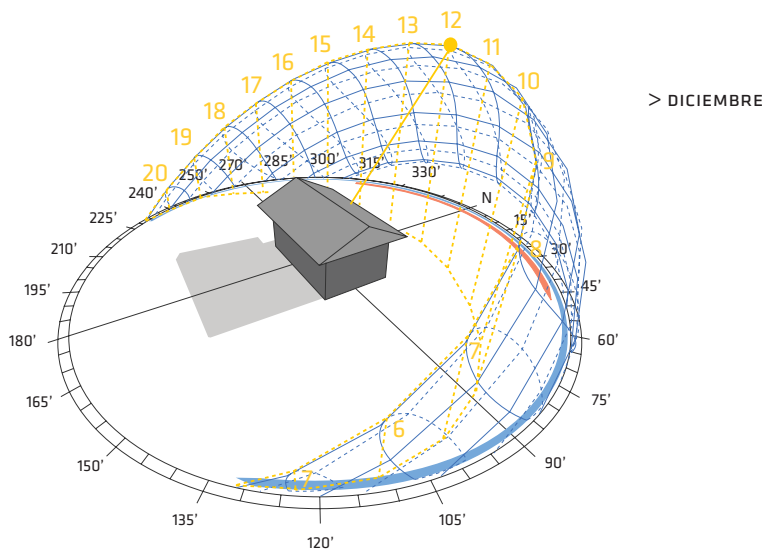
Figura III.3.8.2.1: Posición del sol en solsticio de invierno y verano a las 12:00pm. Sombra proyectada por vivienda ubicada en latitud 53° (Punta Arenas).
