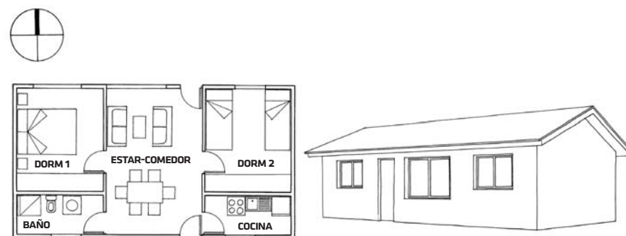
Figura III.3.1: Vivienda 1 piso. 46 m 2 .
