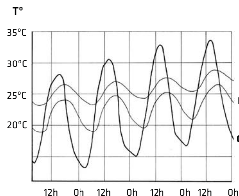
Figura II.1.7.2.2. Curvas de temperatura interior con o sin ventilación nocturna
