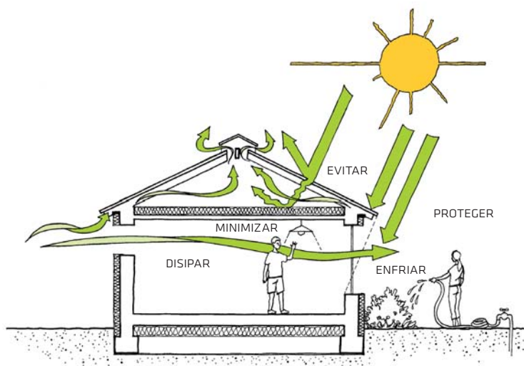
Figura II.1.2: Estrategias generales para periodos de calor.
