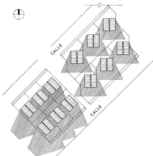
Figura III.2.1.3.1: Flexibilidad de lotes permiten mantener la orientación norte.
