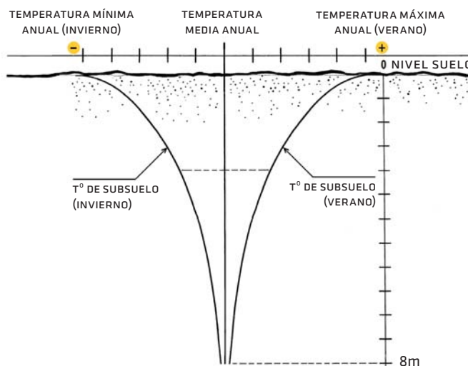
Figura IV.4.2: Variación de la temperatura en el subsuelo.
