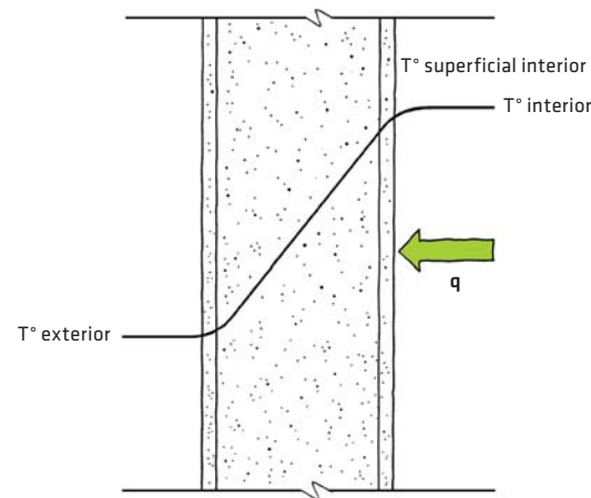
Figura II.1.6.1.1 Perfil de temperatura en muro.
