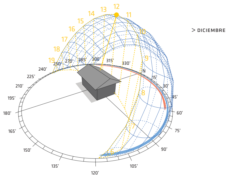
Figura III.3.9.2.1: Posición del sol en solsticio de invierno y verano a las 12:00pm. Sombra proyectada por vivienda ubicada en latitud 34° (El Teniente).
