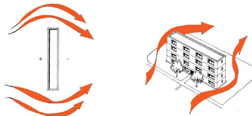
Figura III.2.1.5.3: Presión positiva y negativa de viento generado por un edificio. Facilitación de ventilación natural cruzada.
