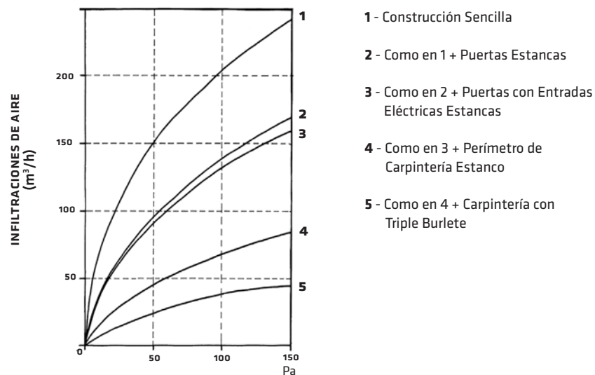
Figura II.1.5.1.6: Efecto en la impermeabilidad de la envolvente con uso de estrategias para evitar infiltraciones de aire.
