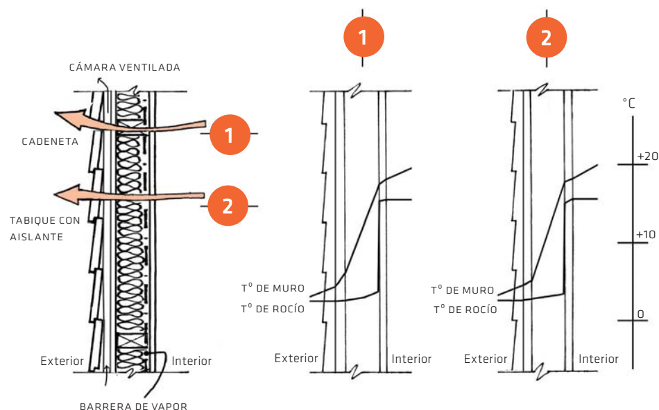
Figura III.3.7.2.4: Riesgo de condensación superficial e intersticial en muro estructurado en madera con 70mm de aislante térmico. Perfil de temperaturas a través de la cadeneta (1) y a través del aislante (2). Análisis realizado en la ciudad de Temuco.
