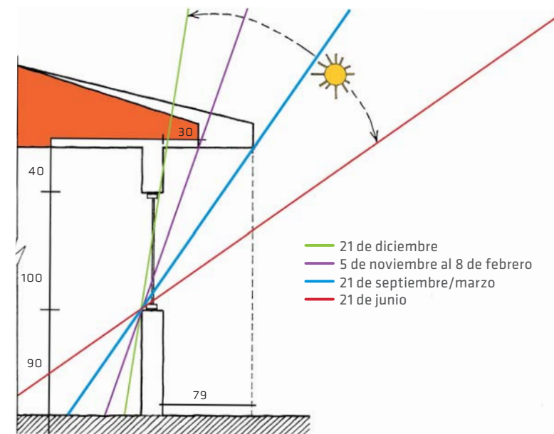
Figura III.3.5.2.3: Dimensionamiento de protección solar horizontal norte para latitud 33° (Santiago).
