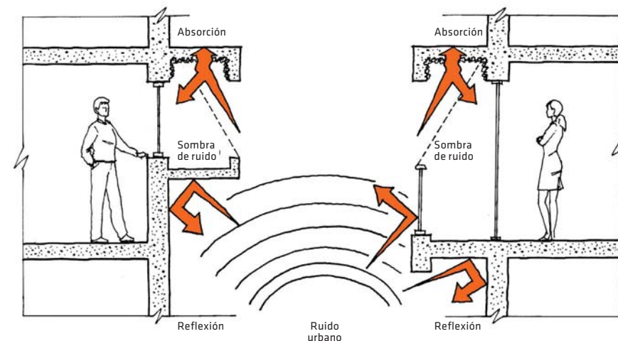
Figura I.5.2.5.2: Aislación acústica de ruido aéreo exterior. Fuente: Ramos (2006).
