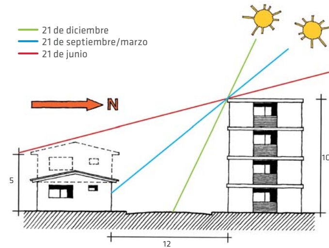
Figura III.3.8.2.2: Sombra proyectada por un edificio de 4 pisos en una vivienda de 1 y 2 pisos ubicada a una distancia igual a 12m entre líneas oficiales. Caso de Punta Arenas.
