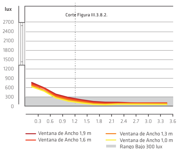
Figura III.3.8.2.6: Niveles de iluminación natural en sección longitudinal de recinto tipo de vivienda social en Punta Arenas, expresado en unidades lux a partir del cálculo de factor de luz diurna.
