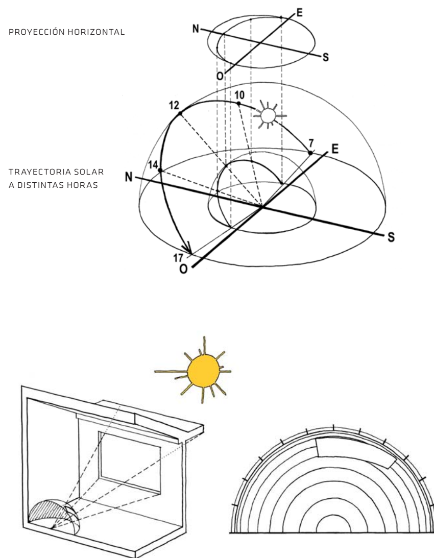
Figura III.2.2.2.2: (arriba) Construcción de una carta solar estereográfica (proyección horizontal de la trayectoria del sol en la esfera celeste para una latitud particular y en todos los días y horas del año; (abajo) Construcción de una máscara de sombra a partir de la carta solar, para una ventana como representación de las obstrucciones sobre un punto de observación.
