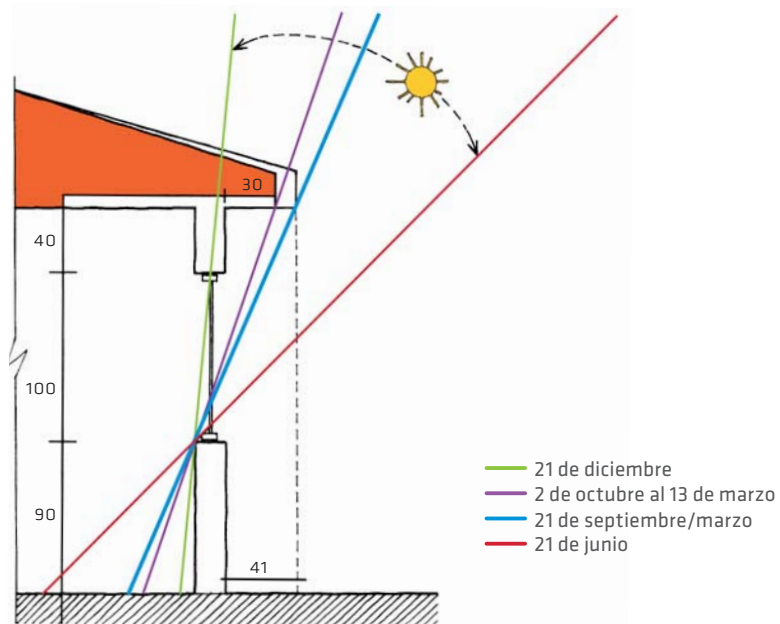
Figura III.3.1.2.3: Dimensionamiento de protección solar horizontal norte para latitud 20° (Iquique).
