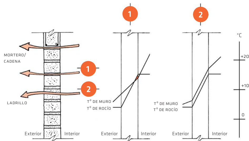
Figura III.3.6.2.4: Riesgo de condensación superficial e intersticial en muro de albañilería de ladrillo, en vivienda ubicada en Concepción. (1) Perfil de temperaturas a través del mortero de pega y (2) a través del ladrillo.
