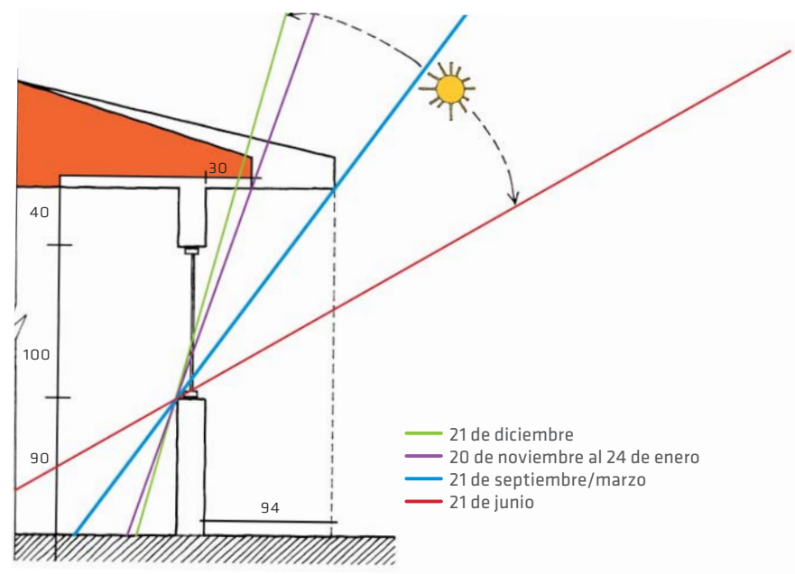
Figura III.3.6.2.3: Dimensionamiento de protección solar horizontal norte para latitud 37° (Concepción).
