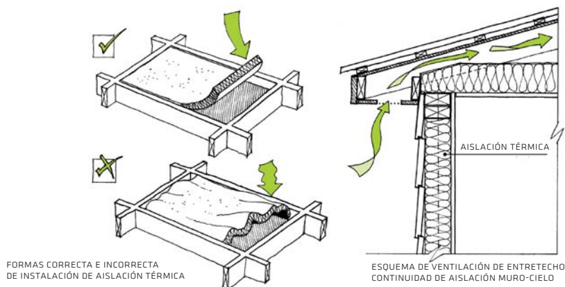
Figura II.1.5.1.2: Aislación térmica bien instalada (izquierda arriba) y mal instalada (izquierda abajo). Caso de aislación térmica bien instalada y continua en encuentro de muro y cielo de la vivienda.
