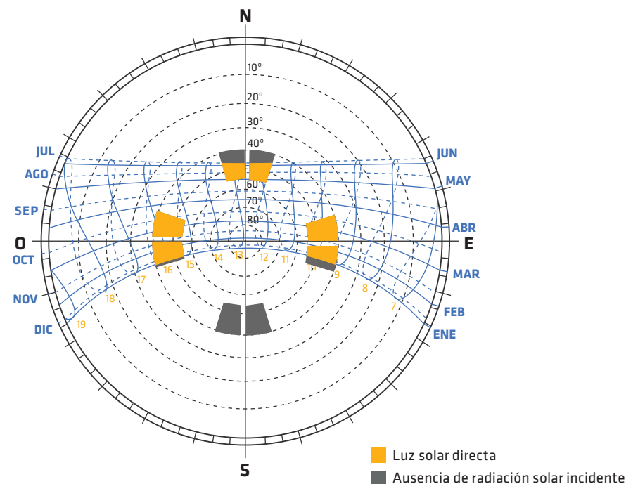
Figura III.3.1.2.5: Carta solar de proyección estereográfica para Iquique. Accesibilidad a la luz solar directa en recinto tipo de vivienda social (3,6 x 2,8 m) a través de una ventana de 1,0 x 1,0 m en las distintas orientaciones.
