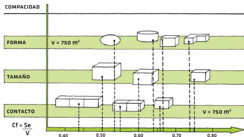
Figura II.1.5.2.1: Variación del coeficiente de forma de un cierto volumen constante.
