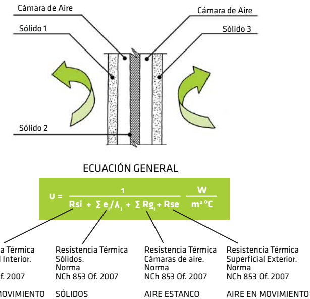
Figura II.1.5.1.1: Ecuación de la transmitancia térmica. NCh 853 Of. 2007
