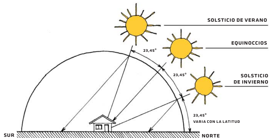
Figura II.1.2.2: Trayectoria del sol (hemisferio sur) respecto de la superficie horizontal terrestre. Vista lateral.
