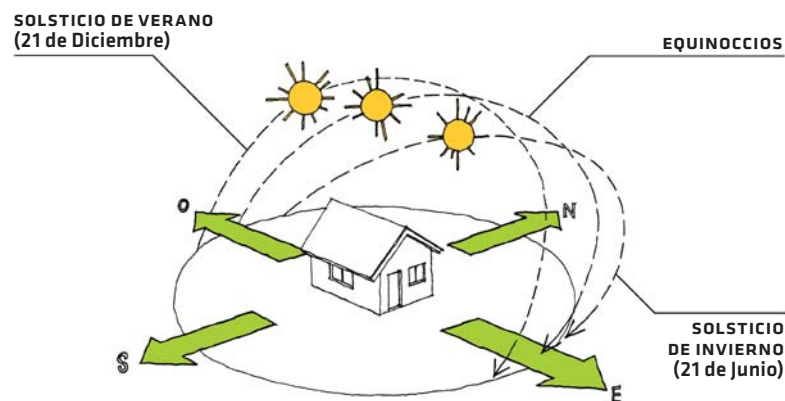
Figura II.1.2.1: Trayectoria del sol respecto de la superficie horizontal terrestre.
