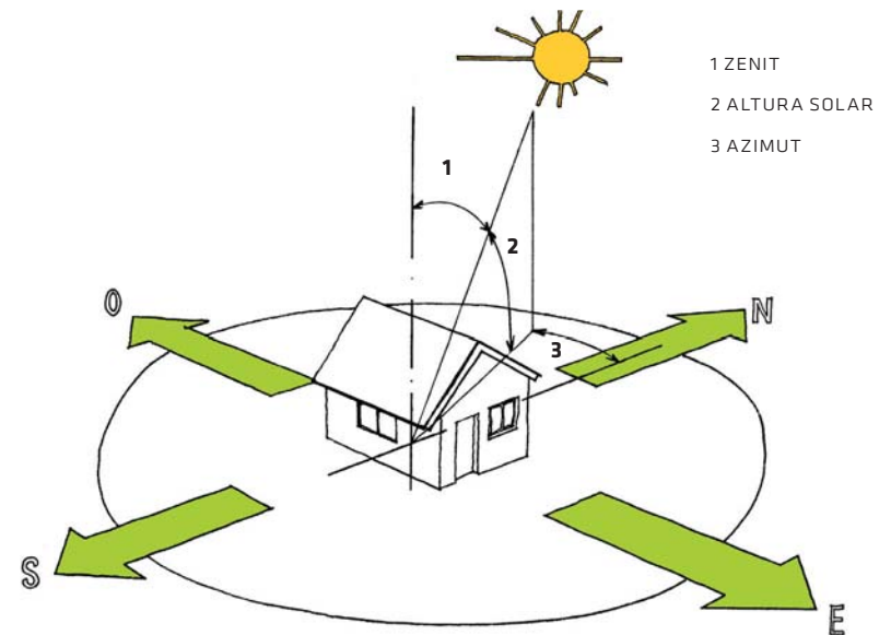
Figura II.1.2.5: Ángulos de posición del sol.
