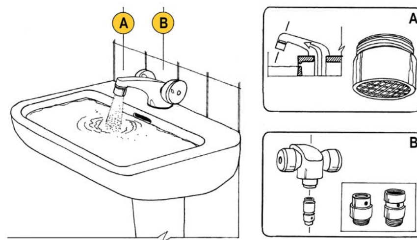
Figura IV.7.1: Aireador de lavamanos (A) y válvula reductora de caudal en ducha (B).
