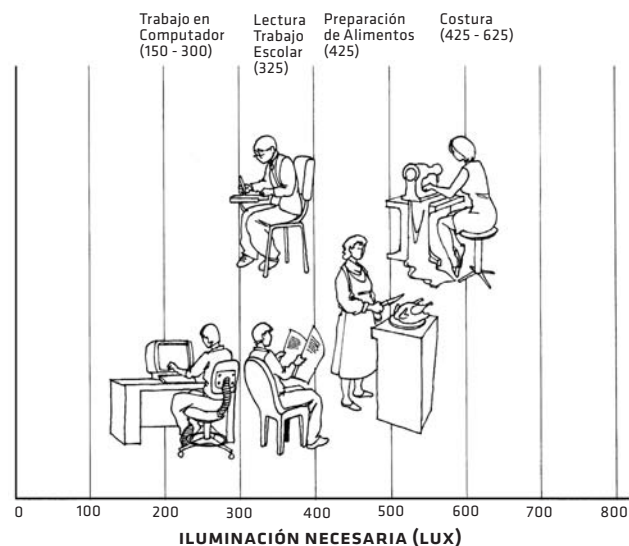
Figura I.5.2.3.1: Confort lumínico de acuerdo a la actividad. Fuente: De Herde, A (2005).
