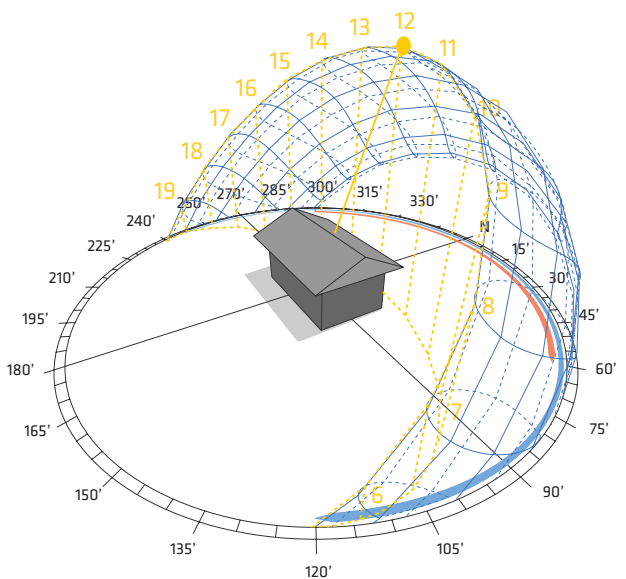
Figura III.3.7.2.1: Posición del sol en solsticio de invierno y verano a las 12:00pm. Sombra proyectada por vivienda ubicada en latitud 38° (Temuco).
