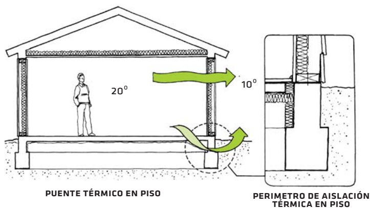
Figura II.1.5.1.4: Puente térmico o pérdida perimetral de calor en piso sobre terreno. Se repara con instalación de aislamiento térmico en el perímetro del piso.
