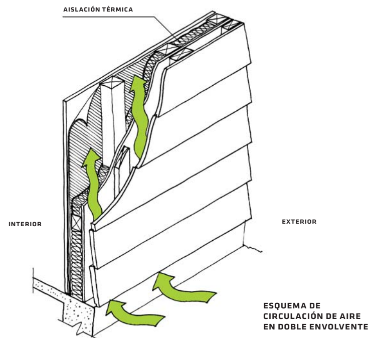
Figura II.1.4.1.12: Muro envolvente de madera (Proyecto FONDEF D03I1020 Centro de Innovación y Desarrollo de la Madera PUC-CORMA).
