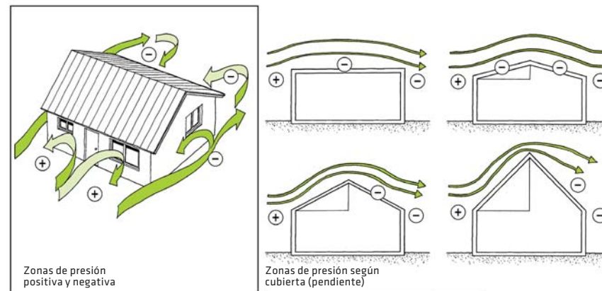
Figura II.1.7.2.3 Flujo de aire alrededor de una vivienda causa presiones negativas y positivas
