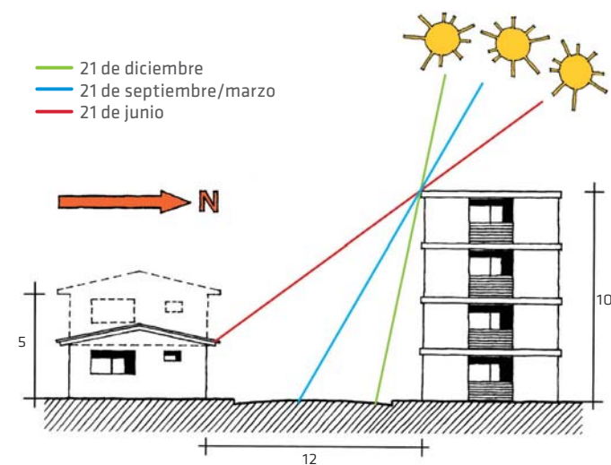
Figura III.3.9.2.2: Sombra proyectada por un edificio de 4 pisos en una vivienda de 1 y 2 pisos ubicada a una distancia igual a 12m entre líneas oficiales. Caso de El Teniente.
