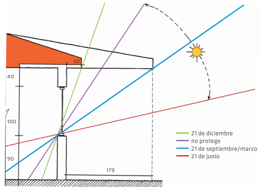
Figura III.3.8.2.3: Dimensionamiento de protección solar horizontal norte para latitud 53° (Punta Arenas)
