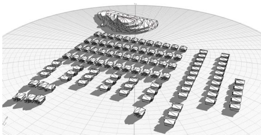
Figura III.2.1.4.2: Estudio de proyección de sombras en conjunto habitacional ubicado en 34° latitud sur. 10 horas. Solsticio de invierno. Se incluye cerro aledaño.
