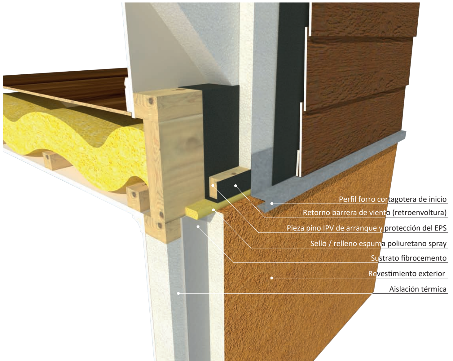
DETALLE 1
