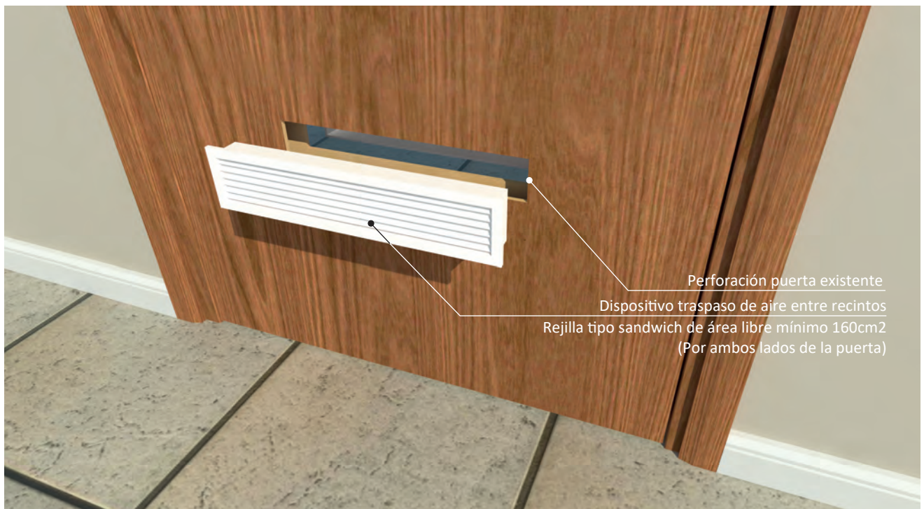
DETALLE 2: DISPOSITIVO DE VENTILACIÓN DE TRASPASO DE AIRE ENTRE RECINTOS
