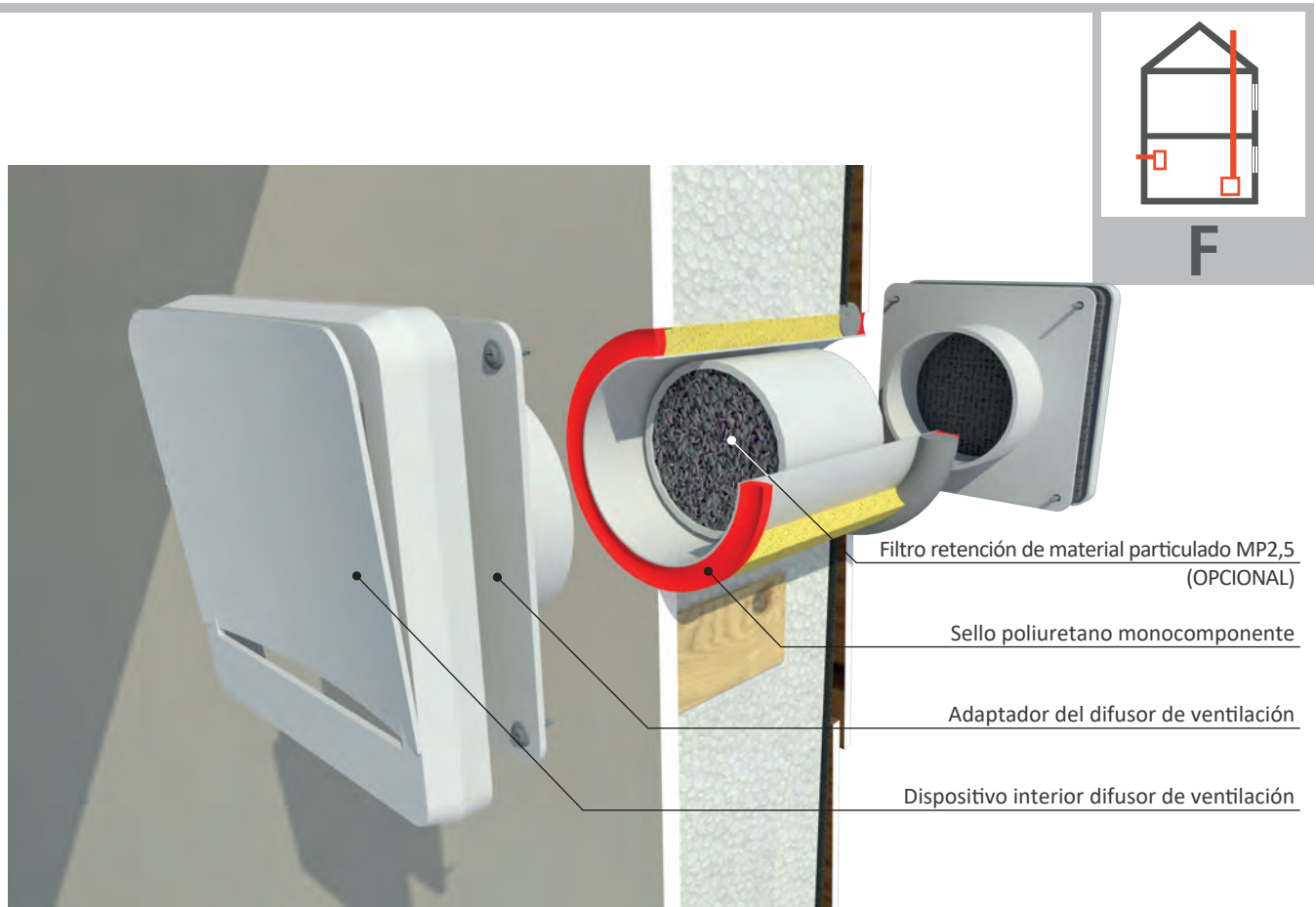
DETALLE 1: DISPOSITIVO DE VENTILACIÓN DE INYECCIÓN PASIVA (Ver también solución HVi1 ó HVi2)
