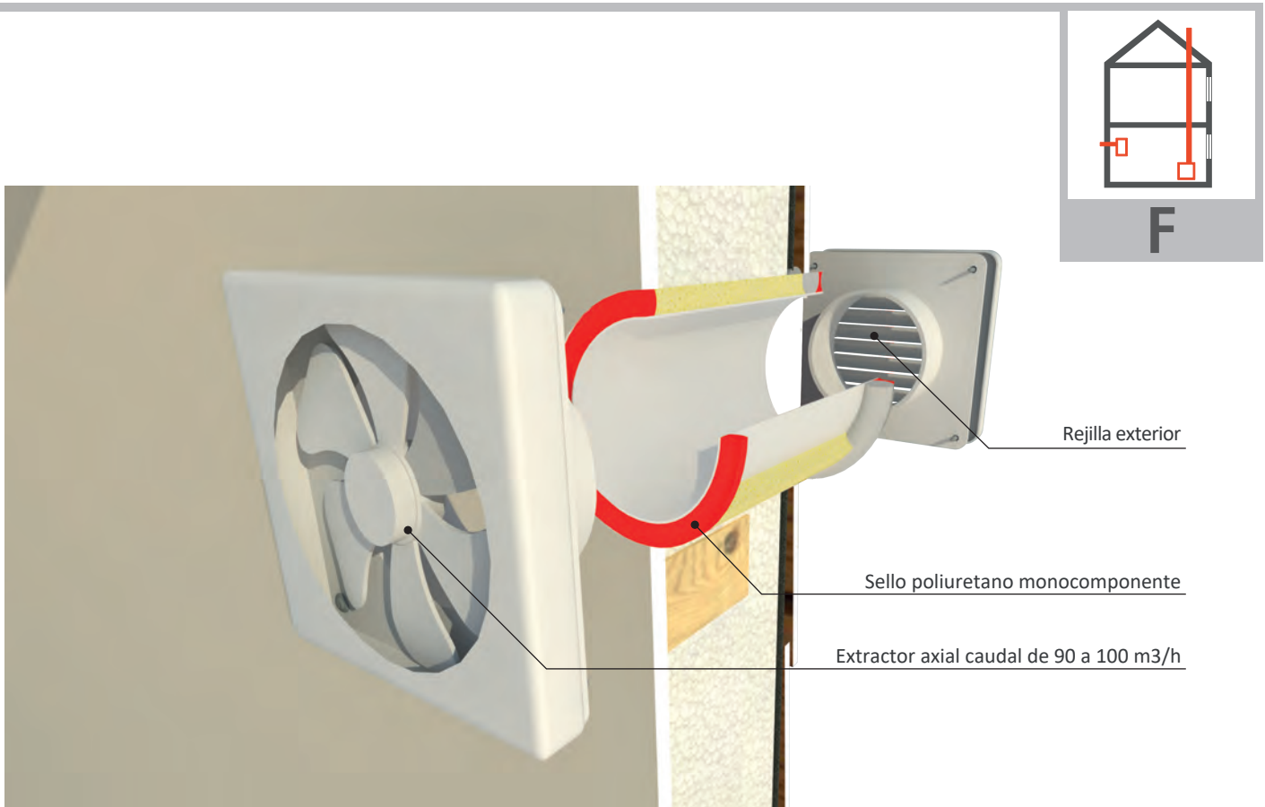
DETALLE 3: EXTRACTOR AXIAL GENÉRICO DE FUNCIONAMIENTO PERMANENTE CON SENSOR DE HUMEDAD REGULABLE, CAUDAL DE 90 a 100 m 3 /h (Ver también solución HVi1 ó HVi2)
